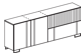
RM1 - 2ANTE 1RIBALTA1CESTO L.2400 P.460 h.903 cod.41MA007 cassa Antracite/frontali Riga-Old Oak cod.41MA017 cassa TortoraST9/frontali TortoraST9-Riga (Mc 0,247)
