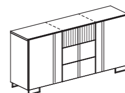
RM7 - 2 ANTE 3 CASSETTI L.1800 P.460 h.903 cod.41MA003 cassa Antracite/frontali Riga-Old Oak cod.41MA013 cassa TortoraST9/frontali TortoraST9-Riga (Mc 0,210)
